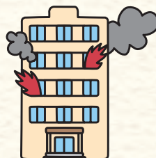
火災・爆発
